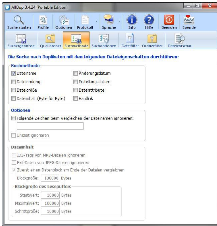
AllDup Suchmethode.
