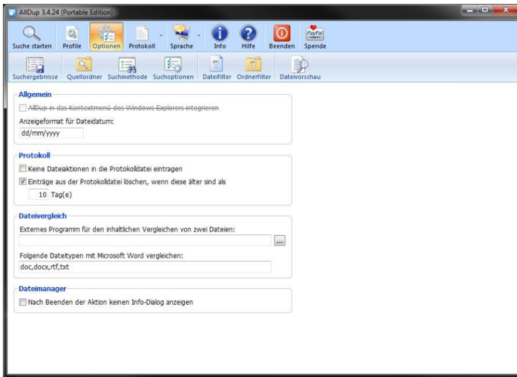
AIDup Programmoptionen.
