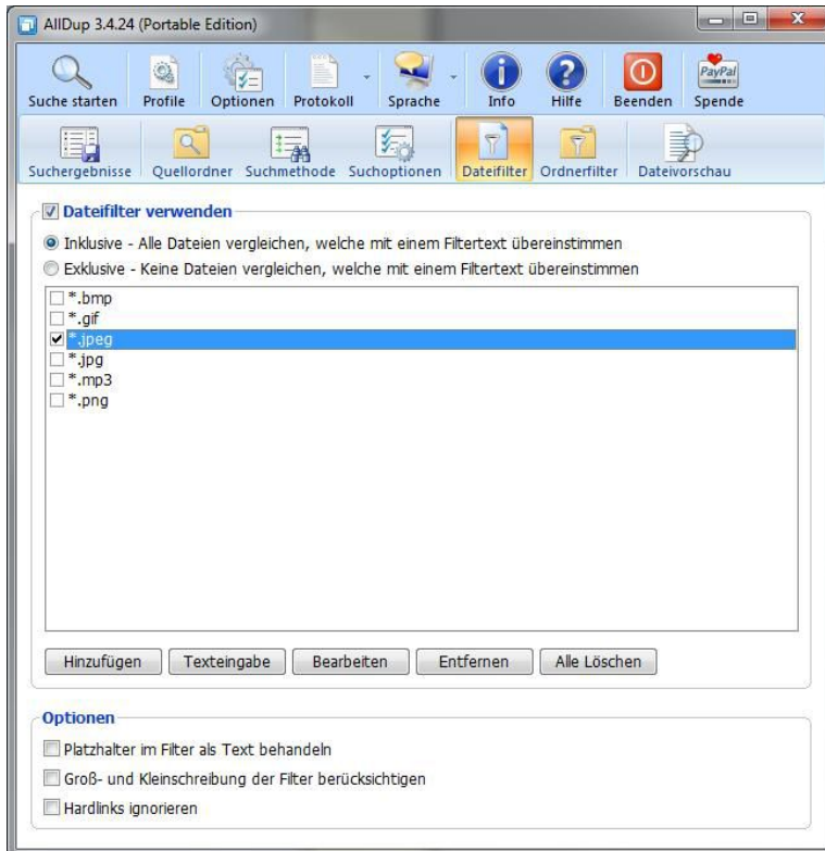
AllDup Ordnerfilter.
