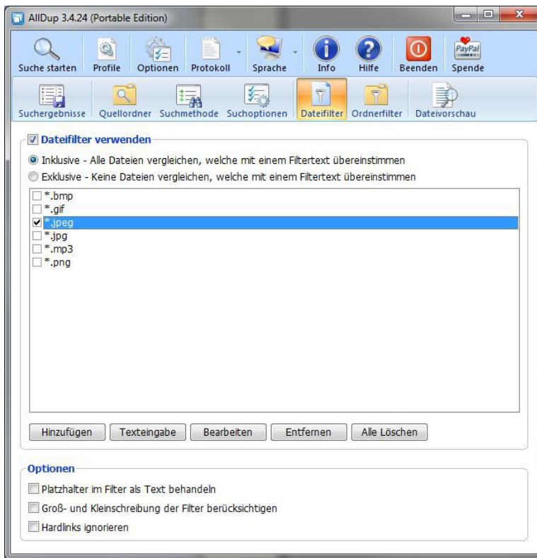
AllDup Dateifilter.
