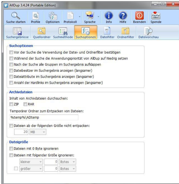
AllDup Suchoptionen.
